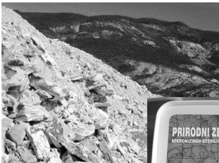
Напазиште зеолита богато тим минералом
